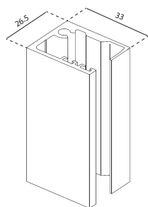
EXPANSOR D-2135
