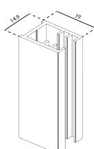
PERFIL PORTAIMÁN U D-2163
