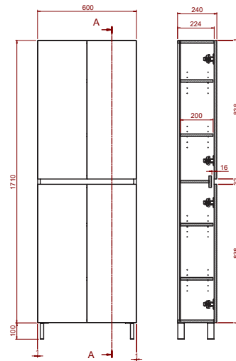
SECCIÓN A-A
