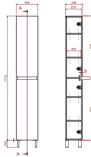
SECCIÓN A-A
